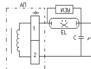
Рис.2 - Электрическая схема
